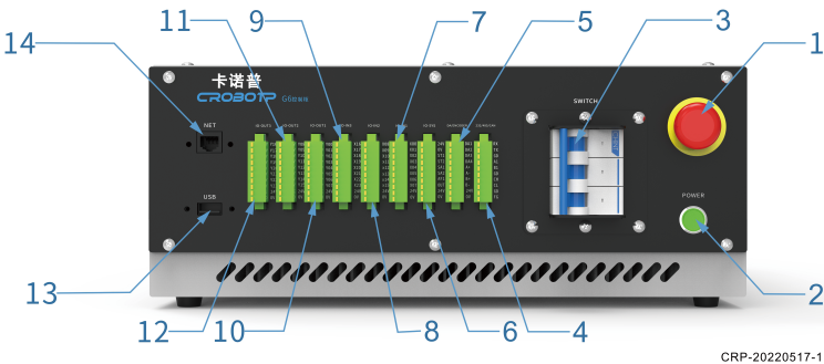
图 3.1 电柜正面接口
