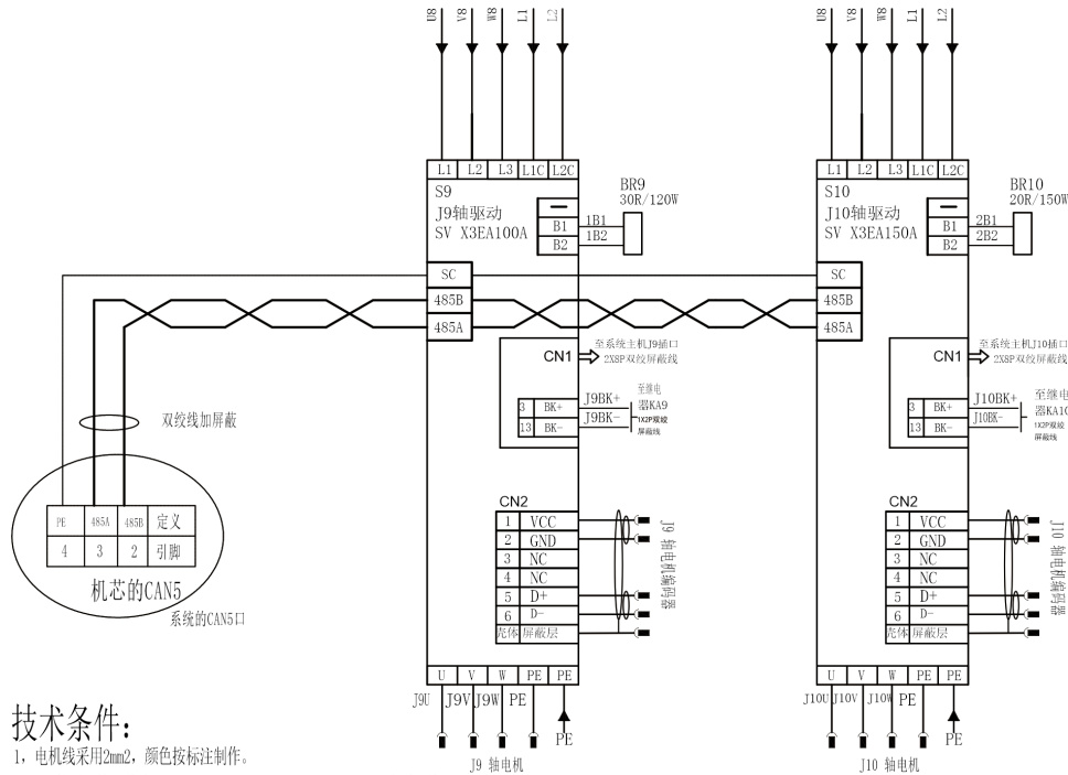
驱动接线图
