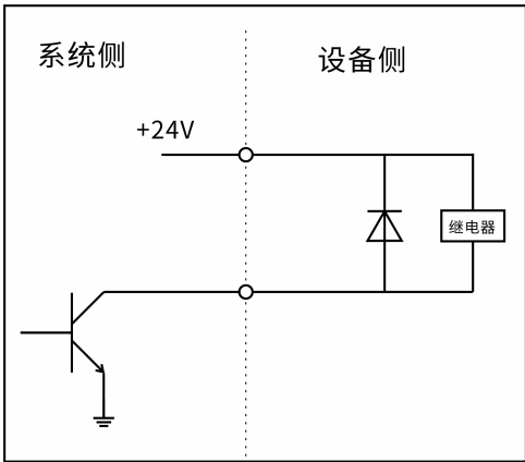
输出接口Y00-Y22原理示意图：
