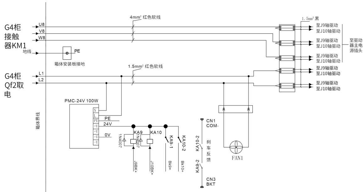
强电原理图
