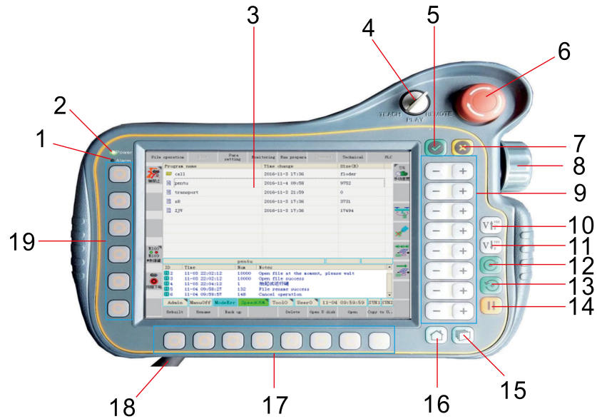
触摸屏示教器正面 (V2)
