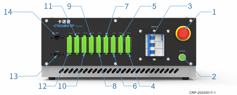
图 3.1.1 电柜正面接口
