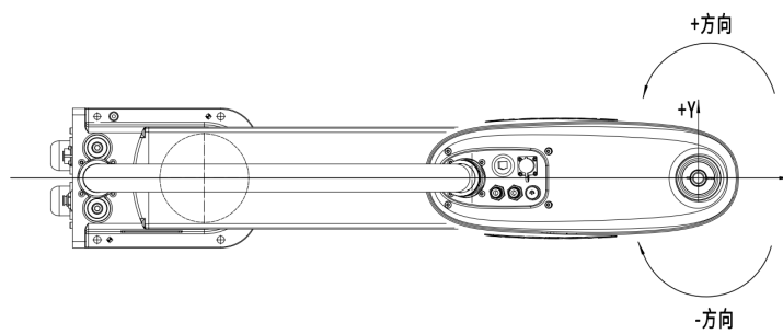
图 6.2.4 第3关节最大行程范围
