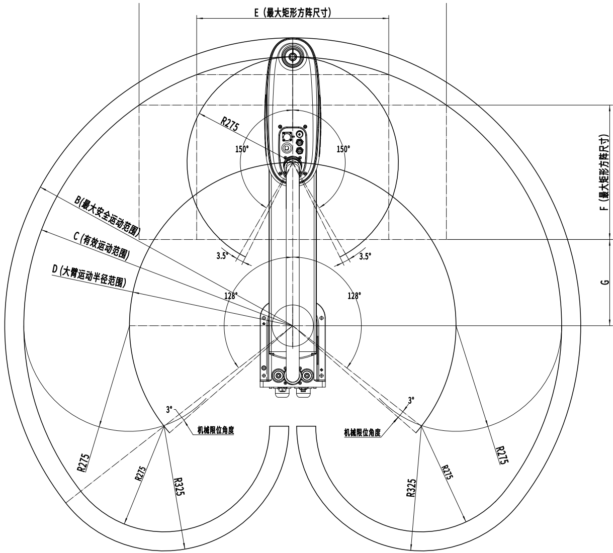
图 4.5 CRP-RS07A-06 标准规格机型运动范围(单位:mm)
