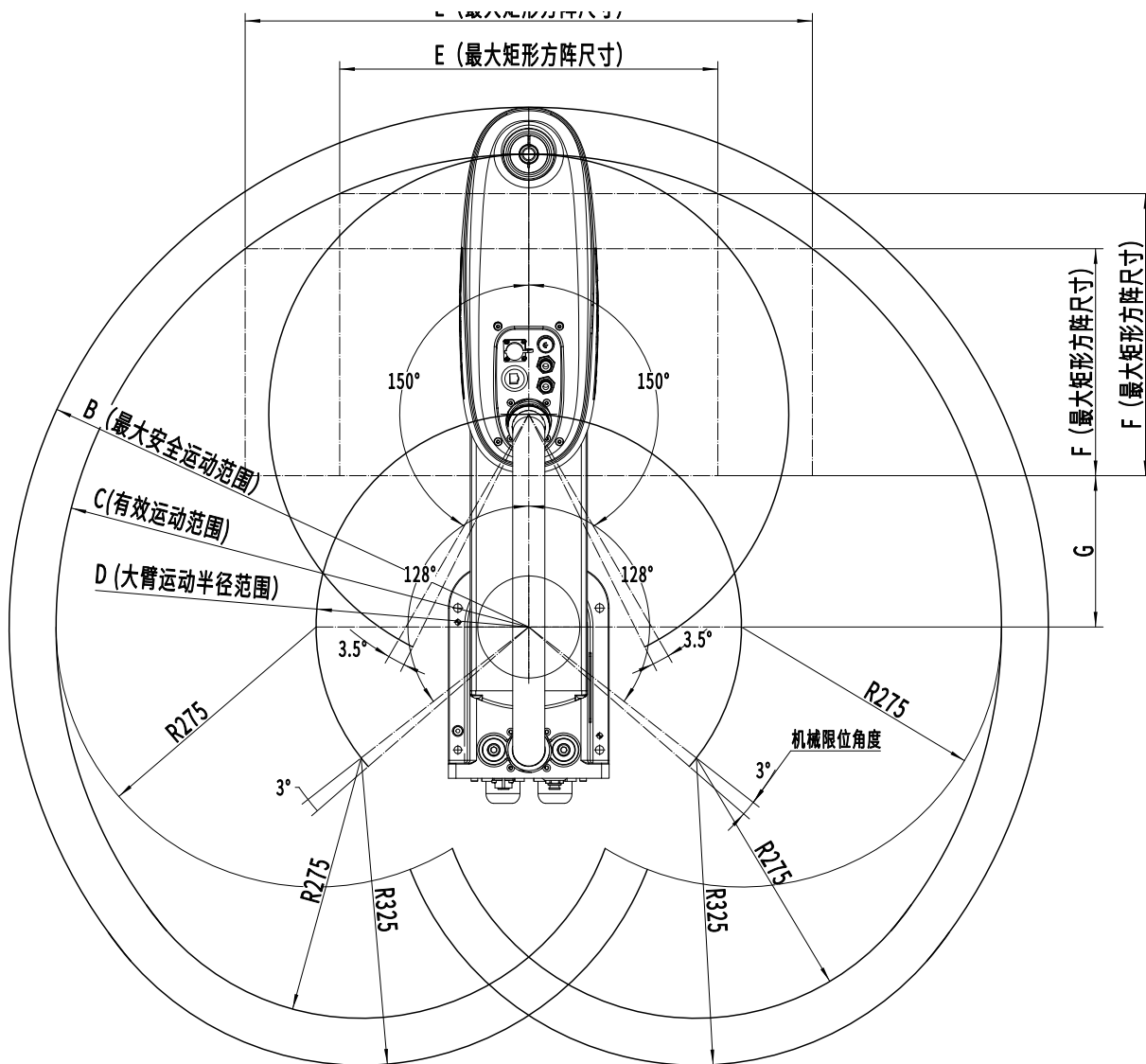
图 4.5 CRP-RS05A-06 标准规格机型运动范围(单位:mm)
