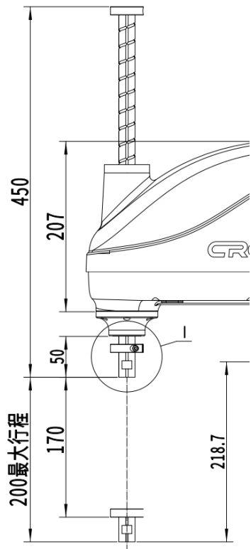
图 6.2.3 第3关节最大行程范围
