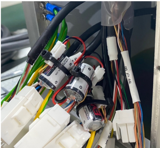
图 5.1.1 电池包更换
