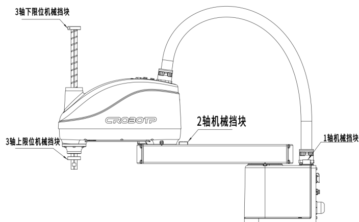
图 6.3.1 机械挡块位置示意图
