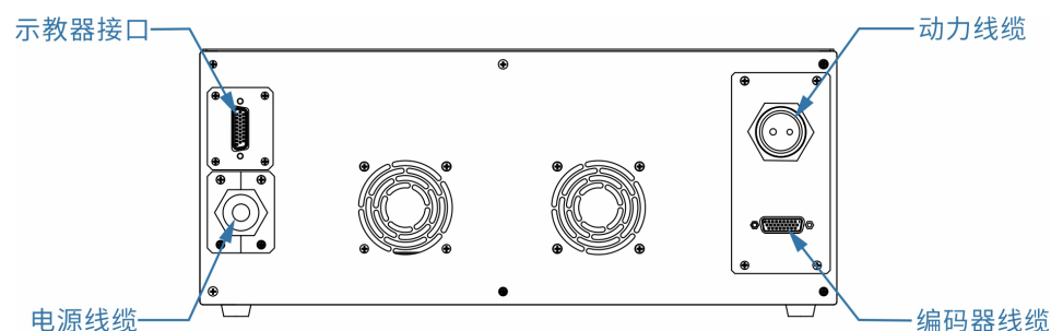
图 3.1.2 电柜背面接口
