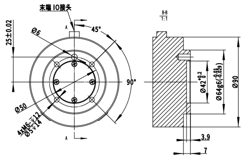
法兰安装图
