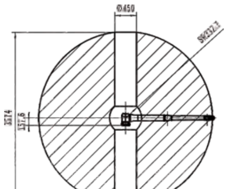
运动范围图
